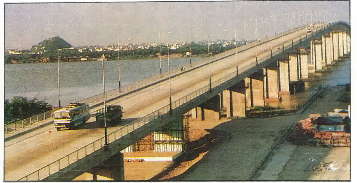
△ 外海大橋。該橋座落在江門外海與中山古鎮之間的滯江河上，全長1769.7米，寬17米，是由香港光大熊谷有限公司承建的。1986年9月1日動工興建，今年5月1日通車。
